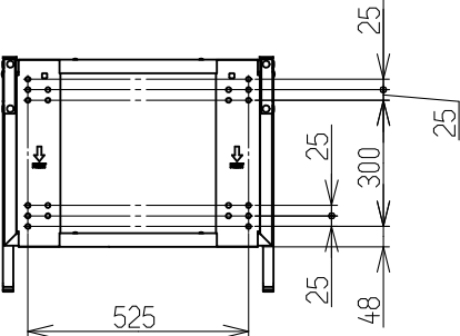
取付穴3種類
